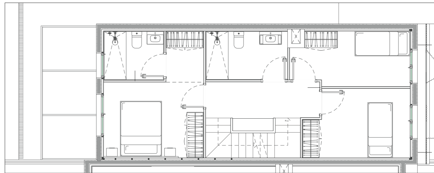
Distribución tipo en planta primera
