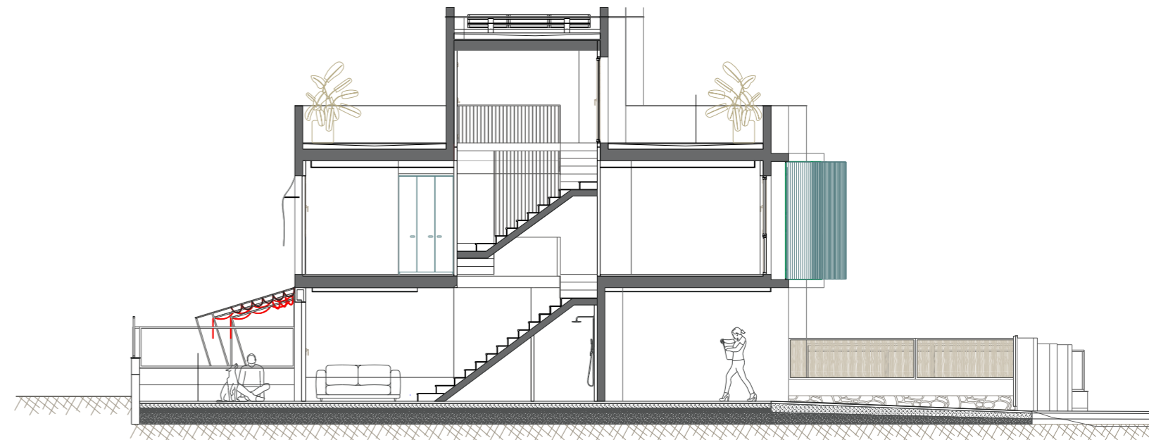
Alzado. Sección vertical
